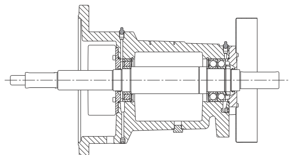
Afb. 31 Lagerstoel met open rollager en dubbele hoekcontactlager die worden gesmeerd via smeernippels
