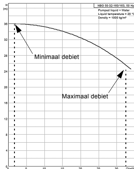
Afb. 6 Voorbeeld uit Grundfos Product Center dat minimaal en maximaal debiet weergeeft
