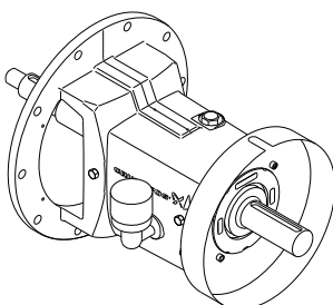
Afb. 21 Lagerstoel met constant-niveau-olievuller
