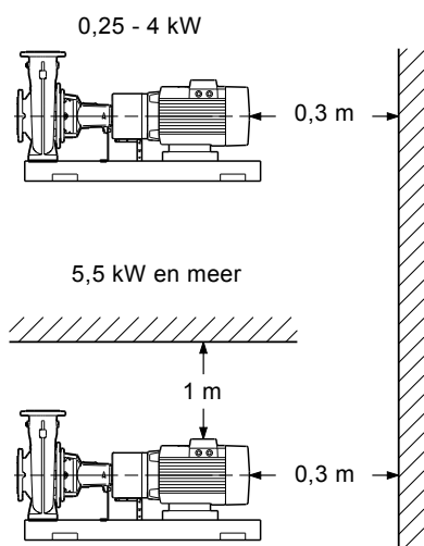
Afb. 7 Vrije ruimte achter de motor
