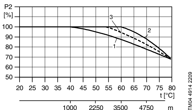
Afb. 4 Het maximale vermogen van de motor hangt af van de omgevingstemperatuur en de hoogte
