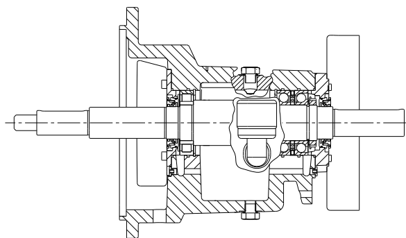
Afb. 34 Lagerstoel met olie-gesmeerde rol- en dubbele hoekcontactlagers
