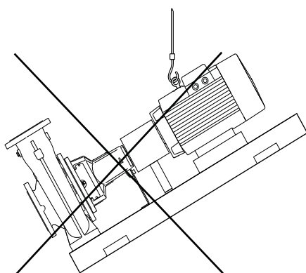
Afb. 2 Incorrect ophijzen van de pomp
