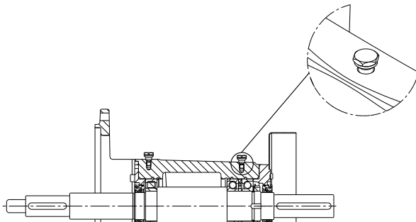
Afb. 24 Lagerstoel met SPM-meetpunten
