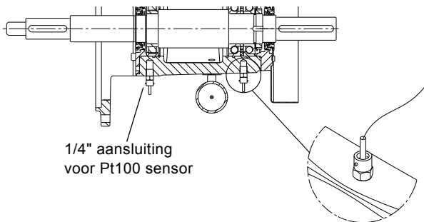
Afb. 26 Pt100 sensoren gemonteerd in lagerstoel
