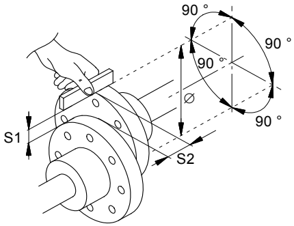
Afb. 12 Uitlijnen
