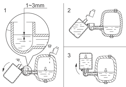
Afb. 22 Vullen met olie
