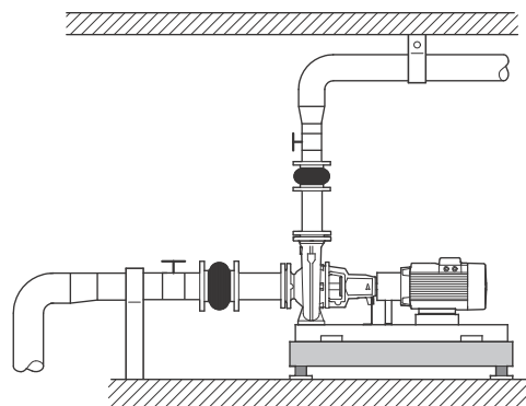
Afb. 14 Bevestiging aan leidingen
