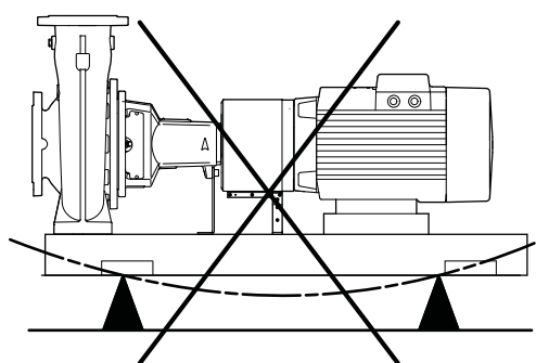
Afb. 10 Incorrecte fundering
