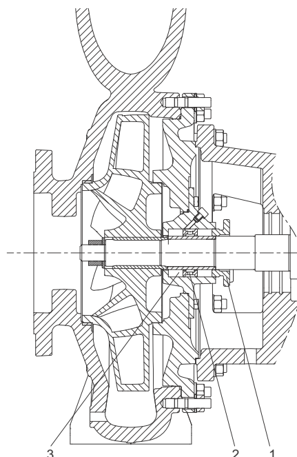
Afb. 29 Dwarsdoorsnede van een stopbuspakking
